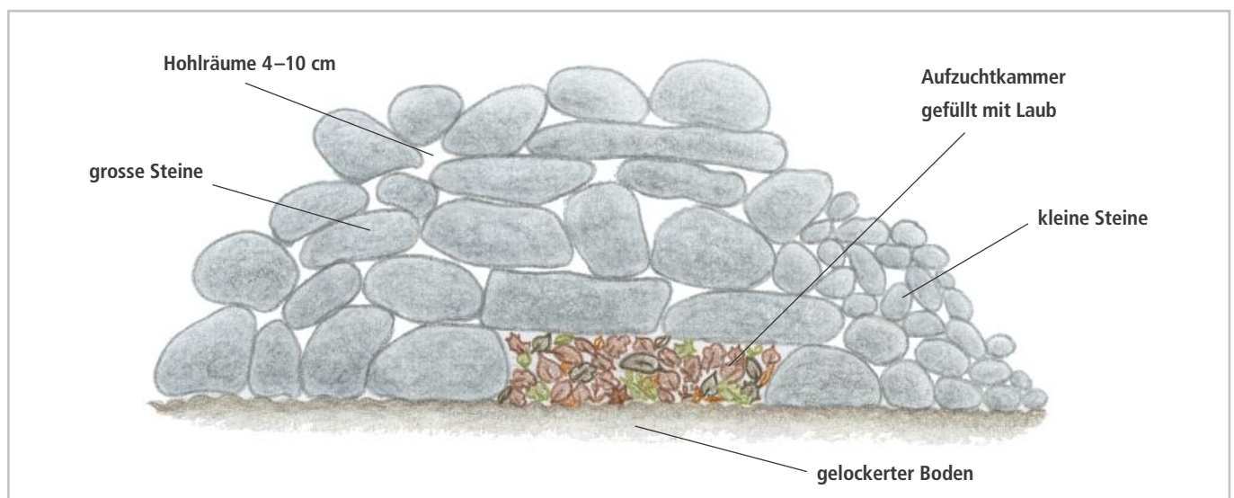
Abb. 15: Aufbau eines frisch erstellten Steinhaufens mit Aufzuchtchamber für Wiesel (Querschnitt). Falls für das Dach der Aufzuchtchamber keine genügend grossen Steine vorhanden sind, kann es auch mit Stammstücken gebaut werden.
