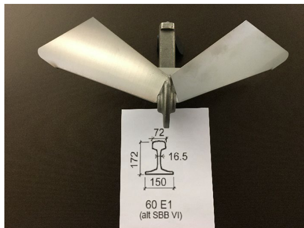
Abbildung 4: Beispiel Amphibienableitblech mit Klemme
