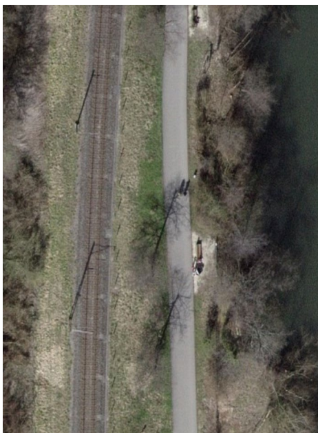
Abbildung 3: Luftansicht der Konfliktstelle in Baden mit einer Passage alle 5 m. Die Konfliktstelle erstreckt sich auf einer Länge von ca. 600 m.
