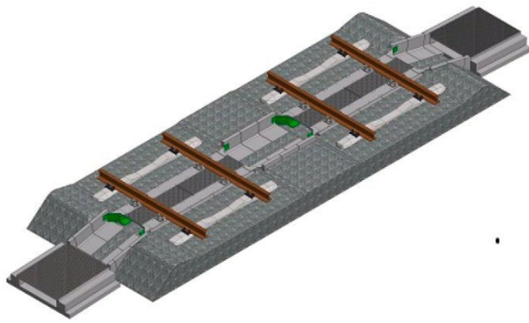
Abbildung 5: 3D Zeichnung der Passage, inklusive der Betonelemente © Movares
